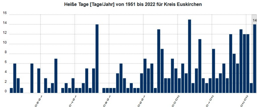
Abbildung 2: Anzahl heißer Tage im Kreis Euskirchen im Zeitraum 1951 – 2022.
