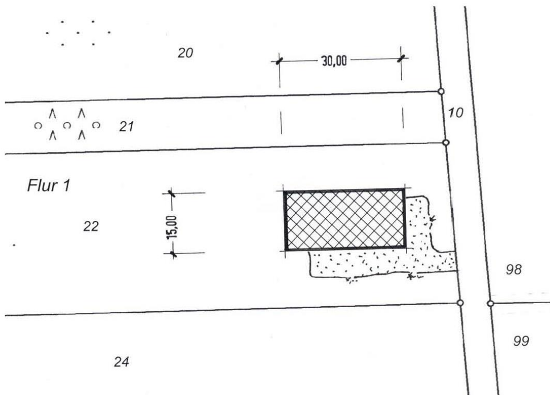
Abb. 1: Lageplan des Bauvorhabens (mit Vermessung)
